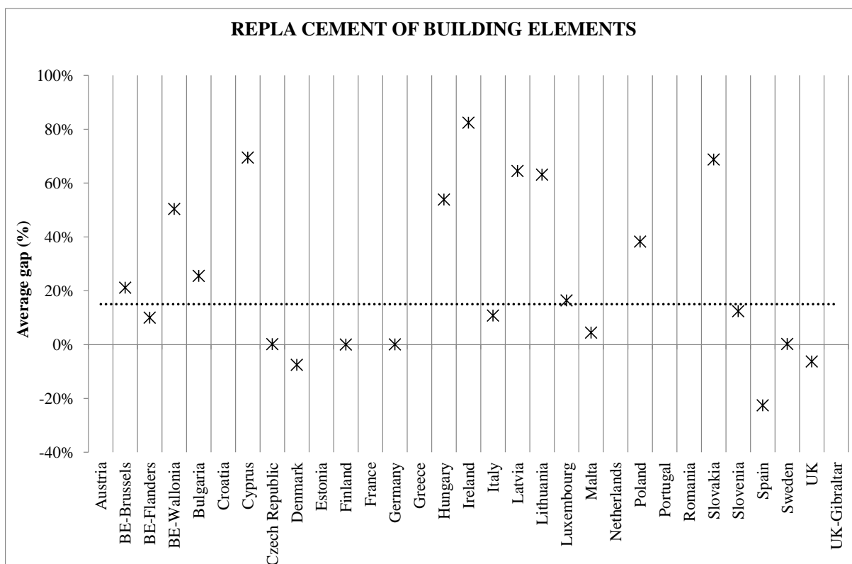
Scarto medio fra i requisiti minimi di prestazione energetica e i livelli ottimali in funzione dei costi: sostituzione di elementi edilizi
