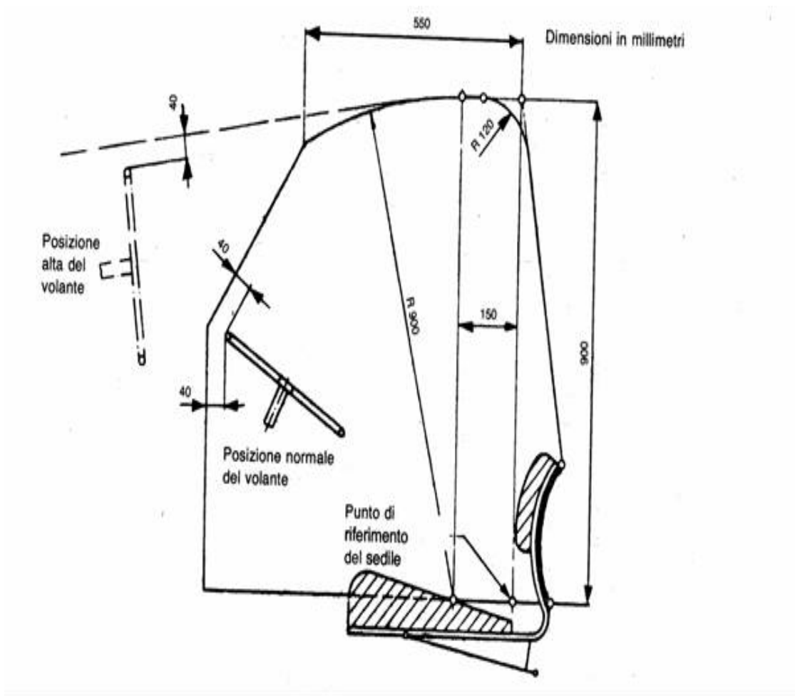
Figura 6 a Vista laterale della zona libera
