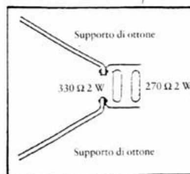
Particolare dei terminali stripline
